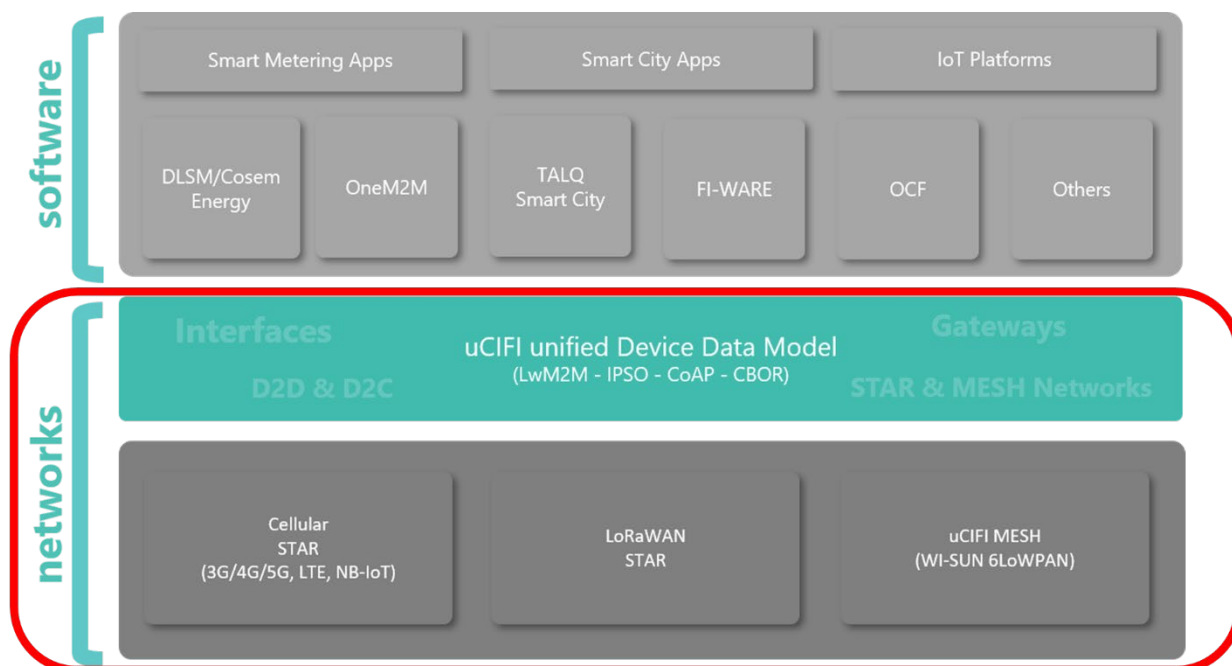
Figura 1. El IoT MAD Lab define los niveles más cercanos a los dispositivos de la Arquitectura IoT.
